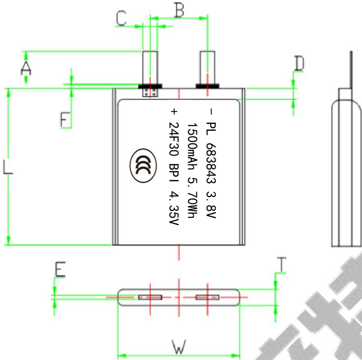
5 电芯图 （单位：mm） Cell drawing (mm)
