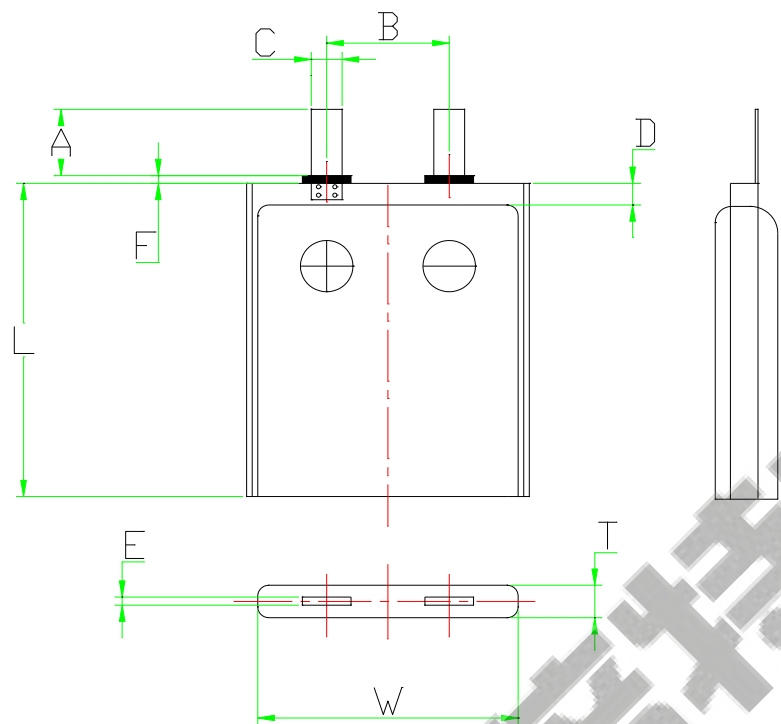
5 电芯图 （单位：mm） Cell drawing (mm)
