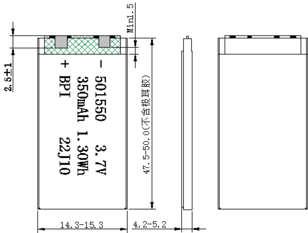
5 电芯图 （单位：mm） Cell drawing （mm）
