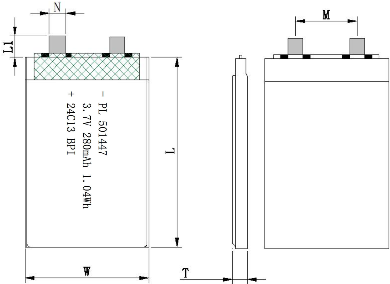
5 电芯图（单位：mm） Cell drawing（mm）
